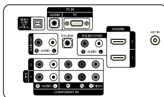
DETALLE DEL PANEL DE TOMAS 3.5"H X 9.0"W
