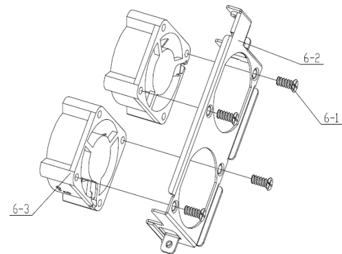
Figure 6 Remove the Fan from Fan rack
