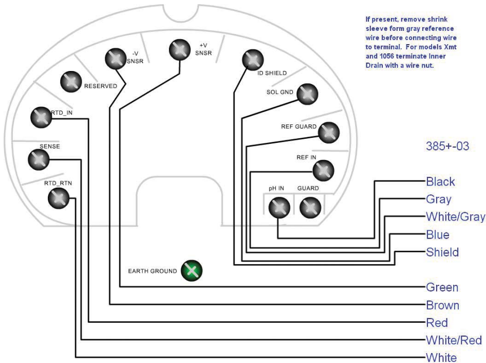
FIGURE 2-7. 6081 VP8 wiring to 385+-03. SMART sensor
