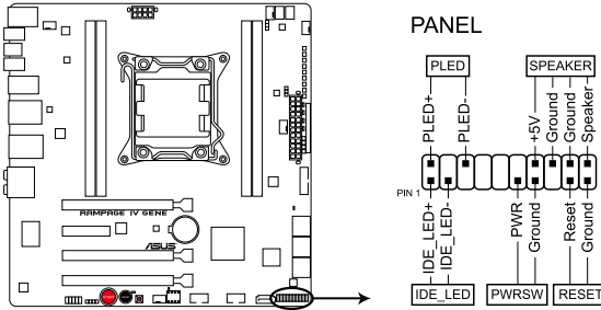
Connecteur panneau système de la RAMPAGE IV GENE
