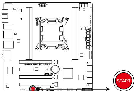
LED d'alimentation de la RAMPAGE IV GENE
