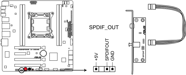
Connecteur audio numérique de la RAMPAGE IV GENE
