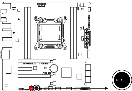
Bouton de réinitialisation de la RAMPAGE IV GENE
