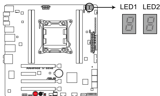
LED de debugage de la RAMPAGE IV GENE
