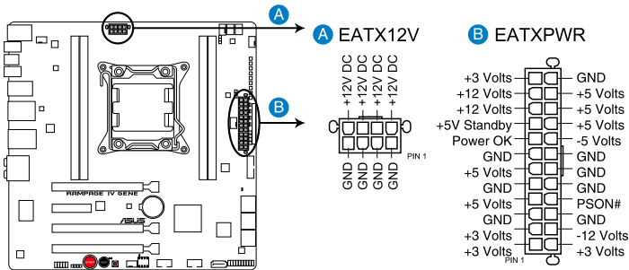
Connecteurs d'alimentation de la RAMPAGE IV GENE
