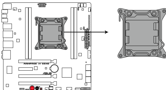
Socket 2011 de la RAMPAGE IV GENE
