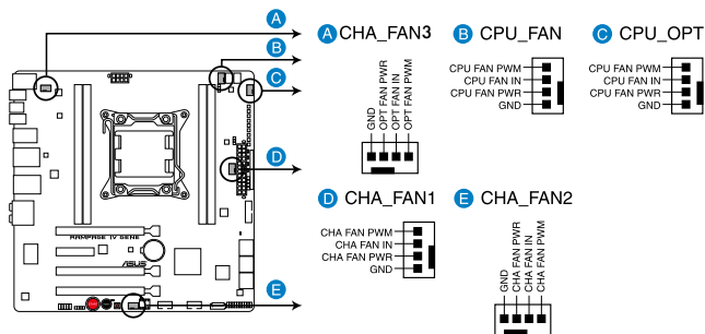
Connecteurs de ventilation de la RAMPAGE IV GENE
