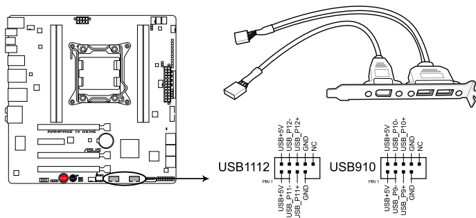
Connecteurs USB 2.0 de la RAMPAGE IV GENE
