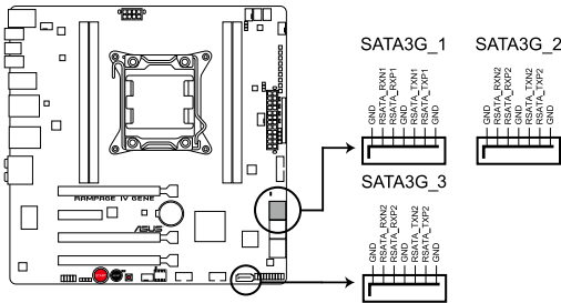
Connecteurs SATA 3Gb/s de la RAMPAGE IV GENE
