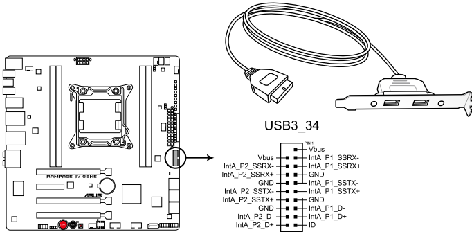
Connecteur USB 3.0 de la RAMPAGE IV GENE
