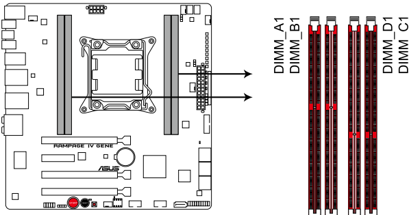
Slots DDR3 de la RAMPAGE IV GENE
