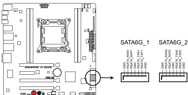
Connecteurs SATA 6.0Gbs Intel de la RAMPAGE IV GENE
