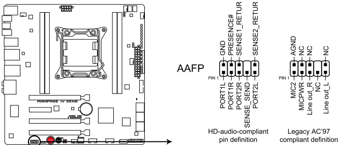
Connecteur audio pour panneau avant de la RAMPAGE IV GENE
