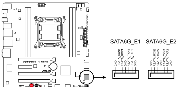
Connecteur SATA 6Gb/s ASMedia de la RAMPAGE IV GENE
